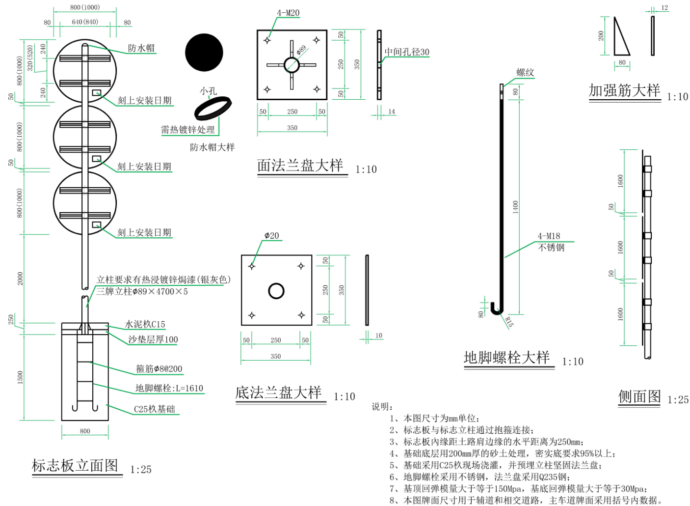
图 2-18 单柱式杆件支撑多个标志大样示例图
